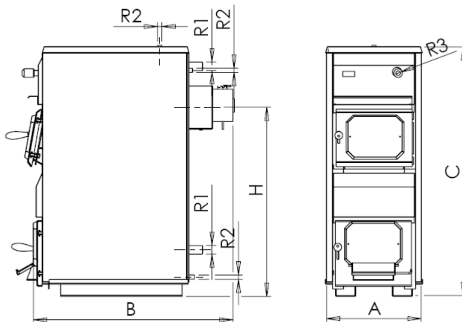
Slika 2. Kotao TKP
