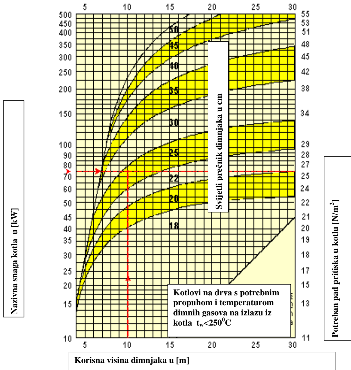
Slika 4 Izbor presjeka dimnjaka kod loženja čvrstog goriva-drvo (Schiedel)
