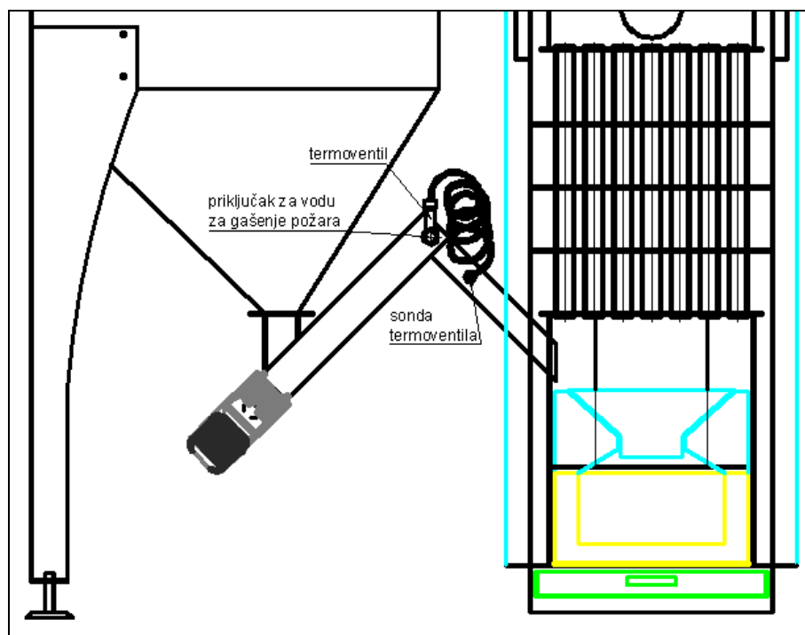
Slika 14. Mjesto priključenja termoventila na sistem za doziranje peleta (PP set)
