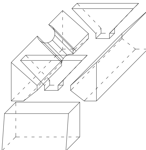
Slika 7. Ugradnja šamota u ložište kotla
