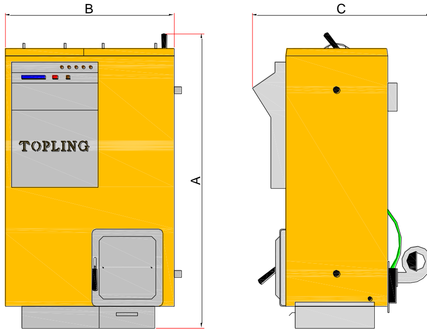
Slika 2. Spoljašnji izgled kotla
