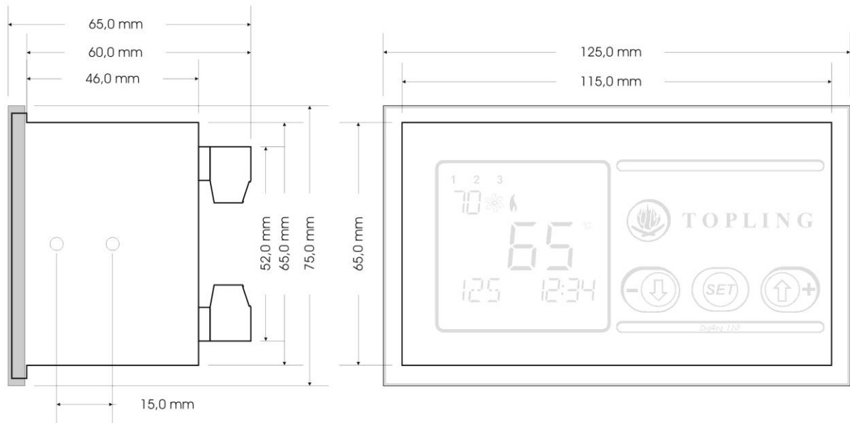
Slika13. Dimenzije regulatora
